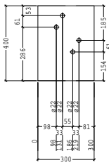
POS 1121 PL400*20 LG 300 AANT. 4
