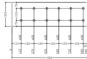
POS 1129 PL300*20 LG 940 AANT. 1
