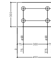
POS 1140 PL300*20 LG 450 AANT. 2
