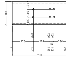
POS 1131 PL300*15 LG 700 AANT. 1
