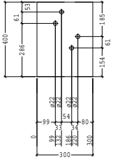
POS 1122 PL400*20 LG 300 AANT. 12
