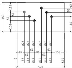
POS 1124 PL350*20 LG 570 AANT. 2
