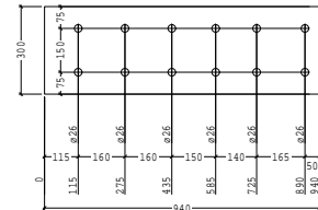
POS 1128 PL300*20 LG 940 AANT. 1
