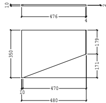
POS 1123 PL350*10 LG 480 AANT. 2
