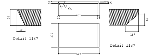
POS 1137 PL300*20 LG 507 AANT. 2
