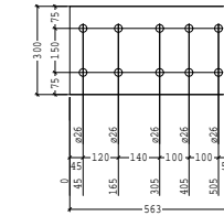
POS 1136 PL300*20 LG 563 AANT. 2
