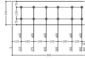
POS 1127 PL300*20 LG 940 AANT. 10
