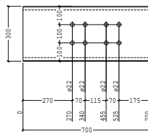
POS 1130 PL300*15 LG 700 AANT. 1
