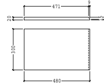
POS 1138 PL300*20 LG 480 AANT. 2
