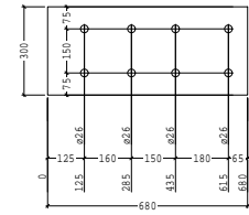
POS 1134 PL300*20 LG 680 AANT. 4
