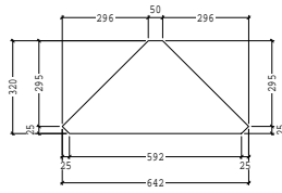
POS 1126 PL320*15 LG 642 AANT. 12
