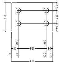
POS 1125 PL350*40 LG 500 AANT. 2
