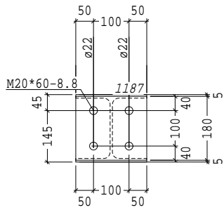
Aanzicht 157, B-B
