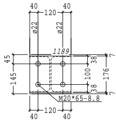
Aanzicht 156, A-A
