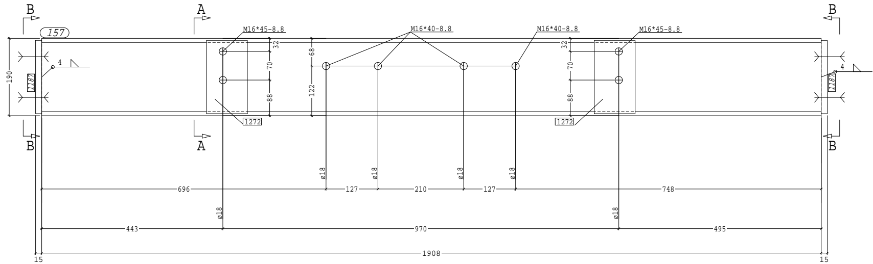
Aanzicht 157, B-B
