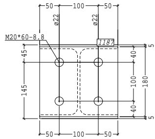
Aanzicht 157, B-B
