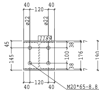
Aanzicht 156, A-A
