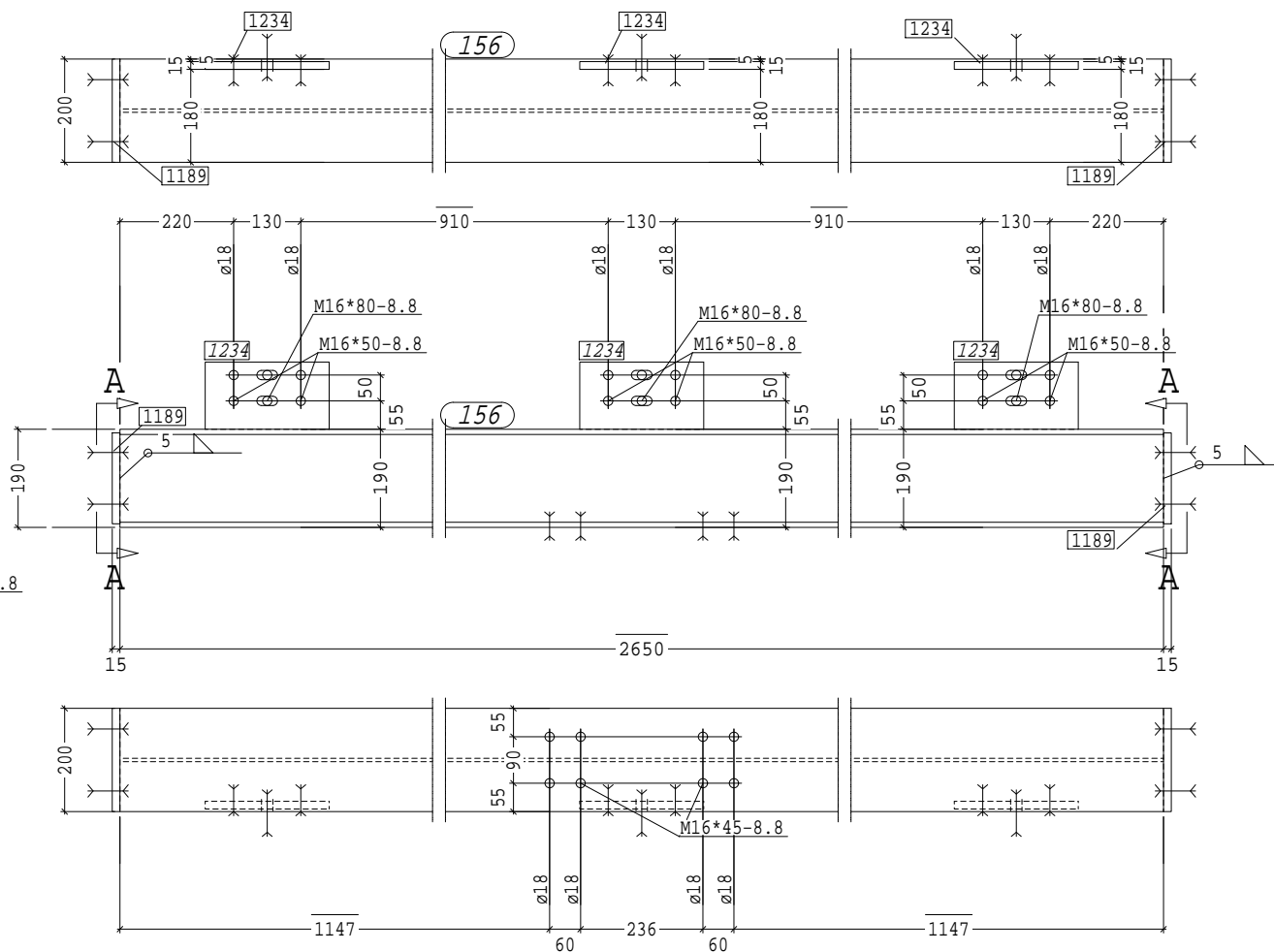
Aanzicht 156, A-A
