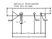
DETAIL TRAPSTRE LENGTE = 800 - BREEDTE = 300 88x UITV.
