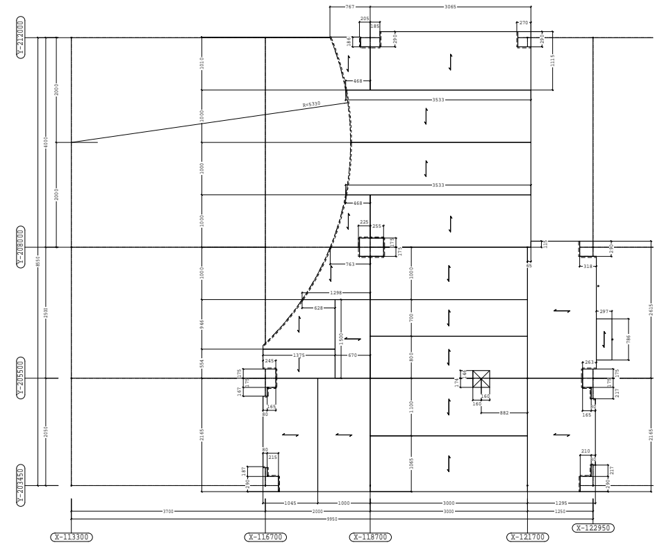
ROOSTERVLOER NIVEAU +6330
