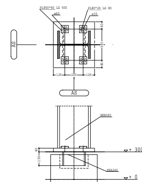
DETAIL VOETPLAAT TYPE 3 2x UITV. ANKERS M30 LEVERING EN PLAATSIING DOOR DERDEN
