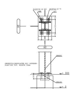
DETAIL VOETPLAAT TYPE 2 2x UITV. ANKERS M30 LEVERING EN PLAATSIING DOOR DERDEN
