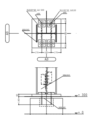
DETAIL VOETPLAAT TYPE 1 4x UITV. ANKERS M42 LEVERING EN PLAATSIING DOOR DERDEN
