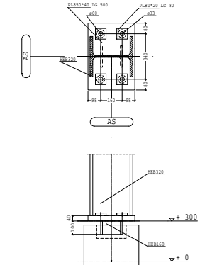
DETAIL VOETPLAAT TYPE 4 2x UITV. ANKERS M42 LEVERING EN PLAATSIING DOOR DERDEN
